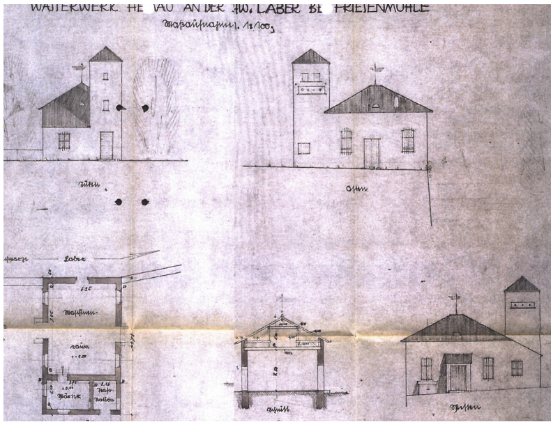
Abb.: Wasserkraftanlage Friesenmühle, Maßaufnahme 1:100, 1952
